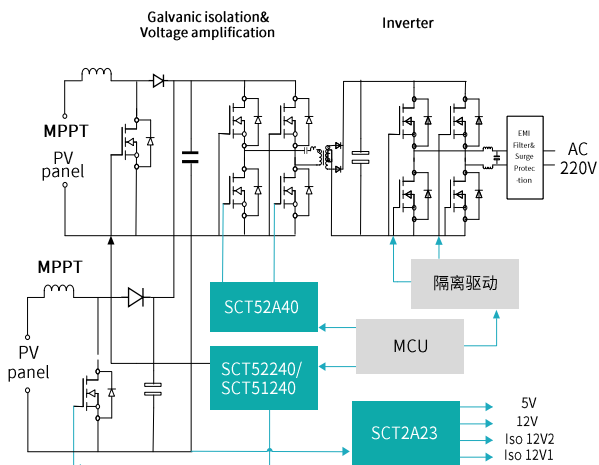
大功率微逆方案
