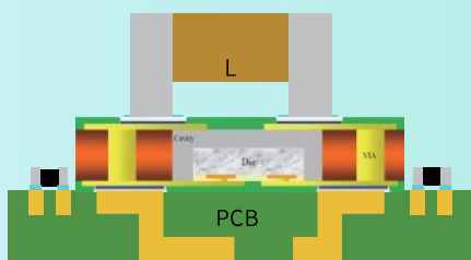
芯洲嵌入式封装模块方案
