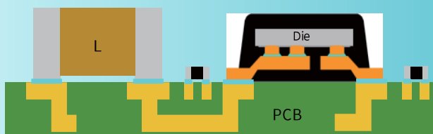
最小分立器件SOT563方案
