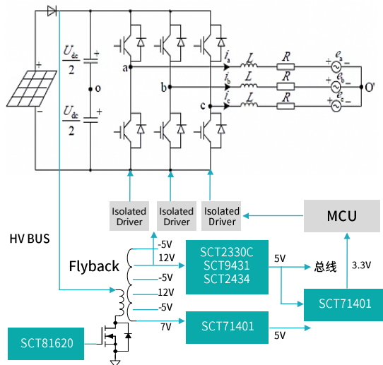
组串式太阳能逆变器
